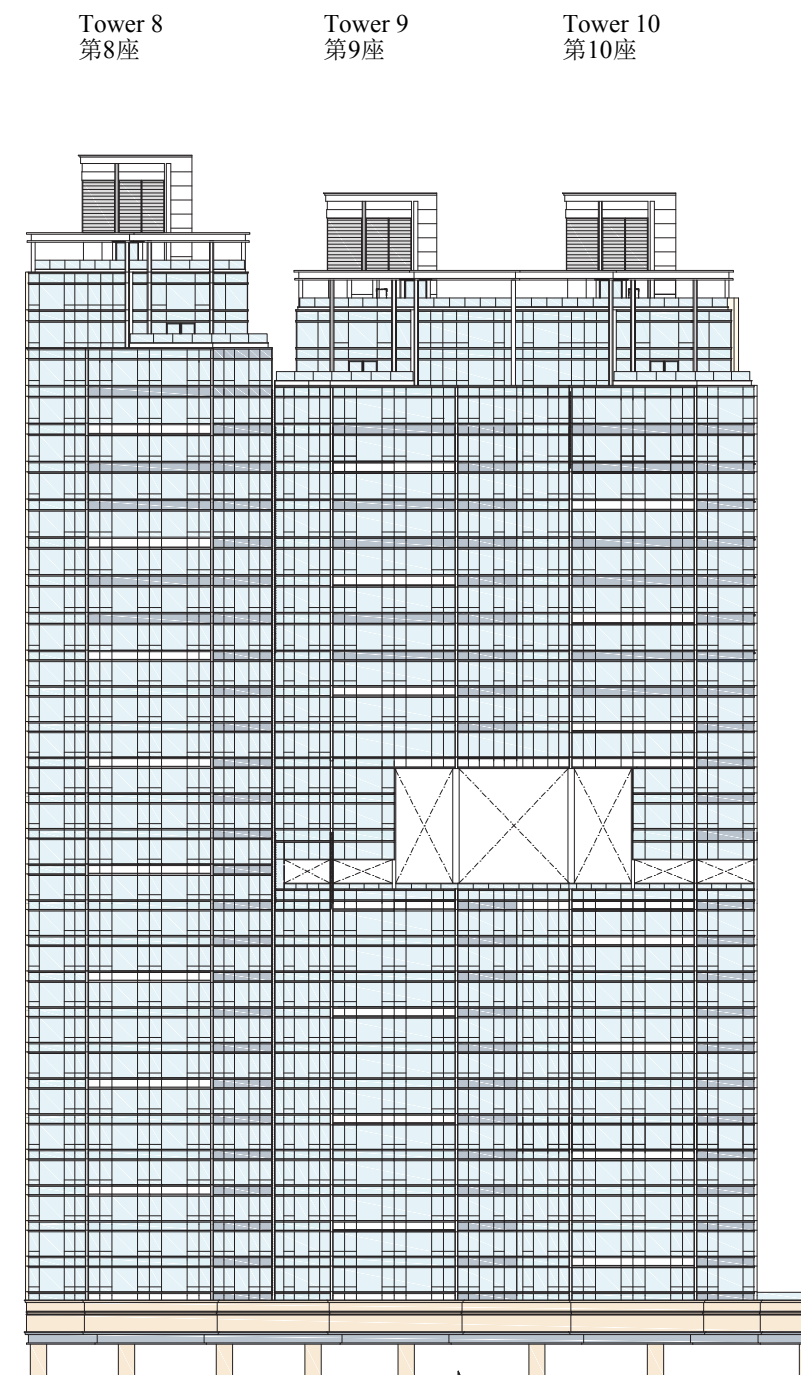
Elevation Plan 4 立面圖 4
